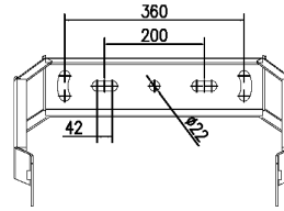
2 Module bracket
