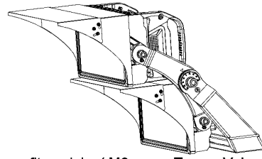
2 Module bracket
